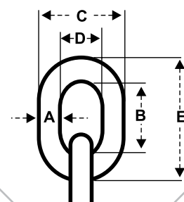
Dimensioni (mm)
